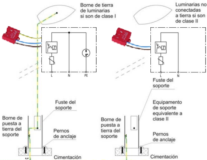
Esquema extraído de la guía BT-09 sin representación de los conductores activos y con DEHNcord incorporado.
