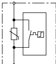
Esquema del V SCP 1 300
