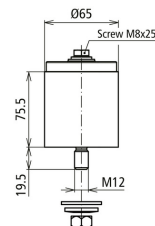
Dimensiones del V SCP 1 300
